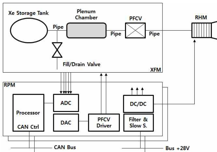
그림 1. 차세대 소형위성 RJT 시스템 구성(안)
